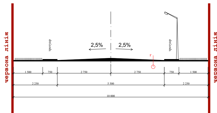
Розріз 1-1
