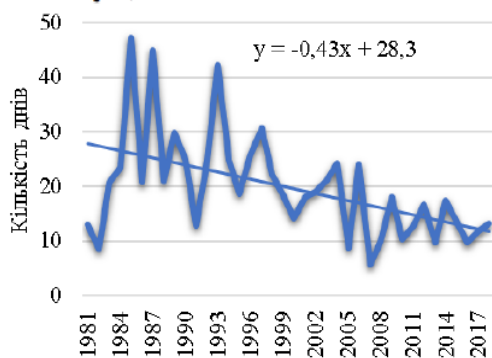
Кількість днів з мінімальною температурою нижче 5 перцентилі T мін
