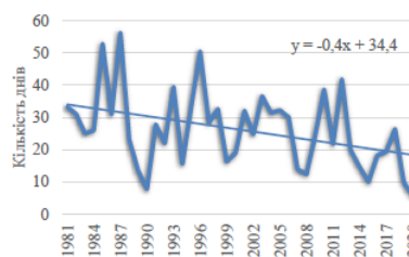
Кількість днів з T мін < -20,0°C
