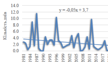
Кількість днів з T мін < -20,0°C
